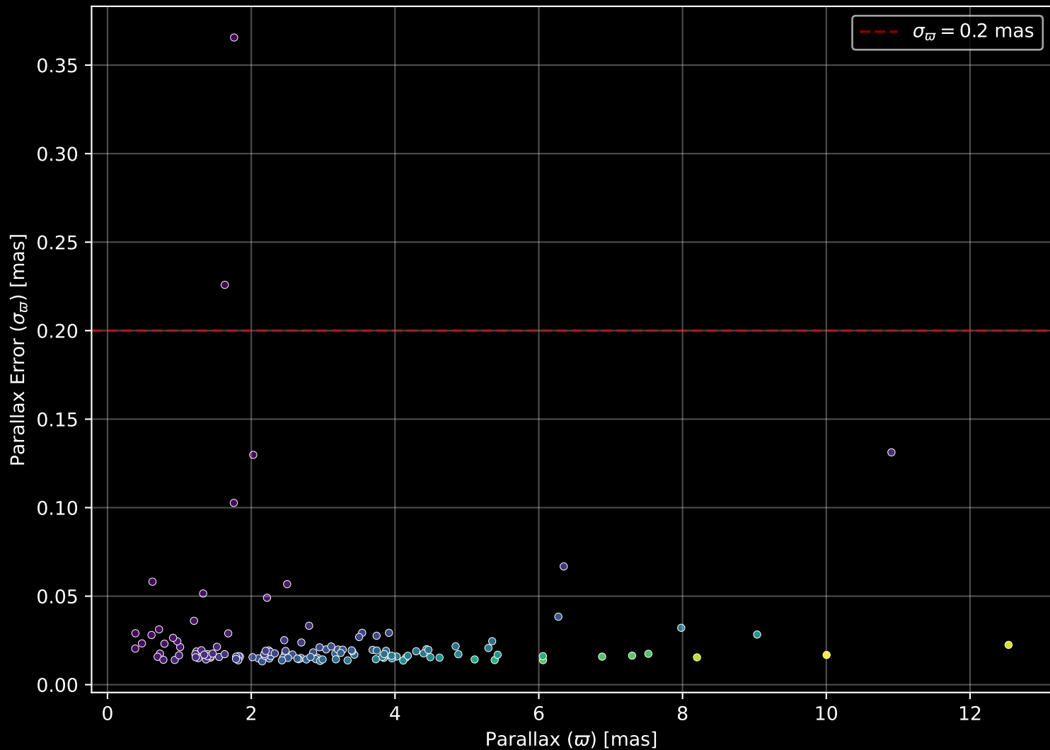
GALAH DR4 Field: [6596] Parallax Quality (n= 131)
