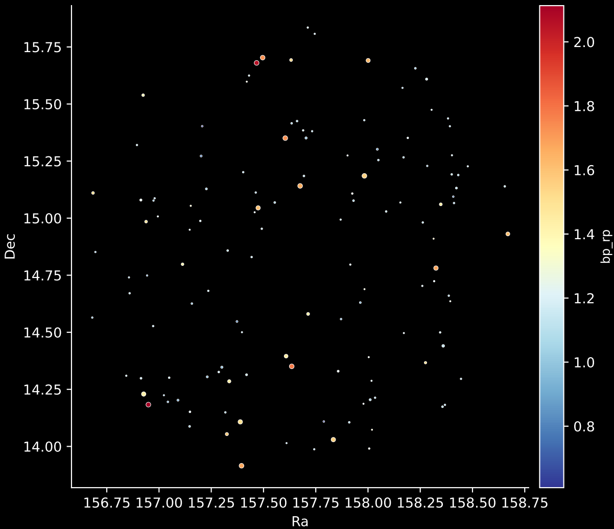
GALAH DR4 Field: [6596] Stars: 131
